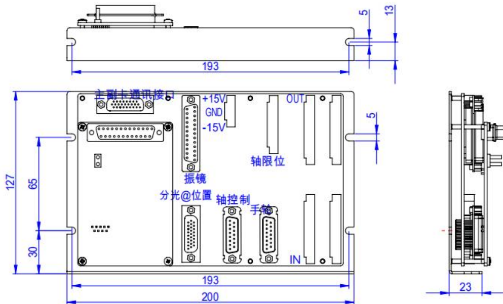
PCIE 主卡
